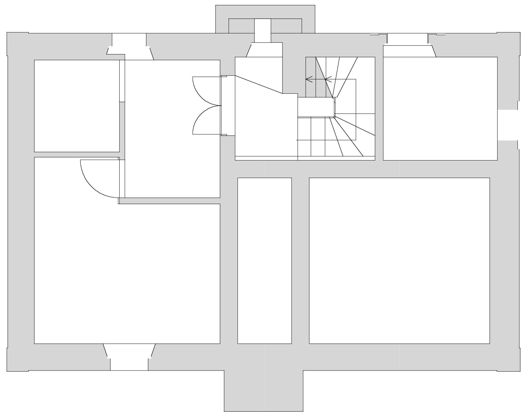
Grundriss Untergeschoss
