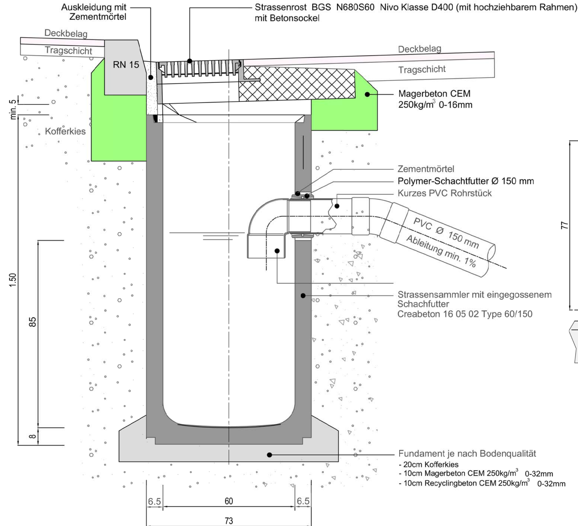
Schnitt A-A
