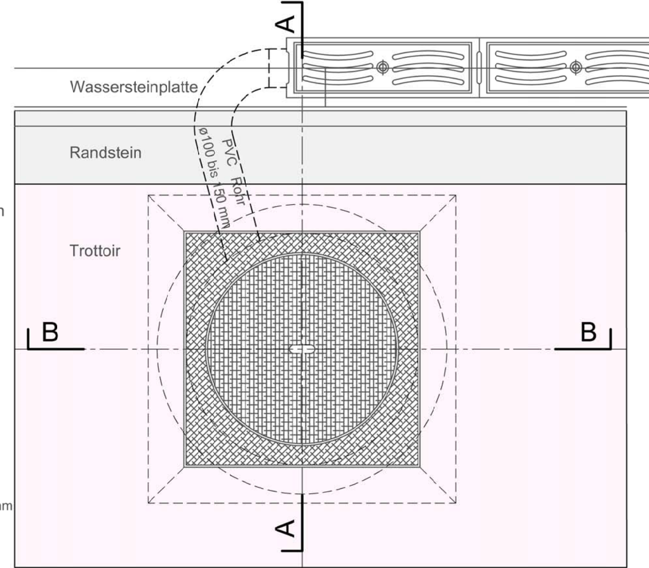
Grundriss
